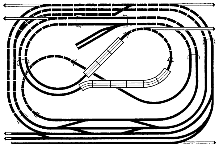
Gleisbild Grundanlage
